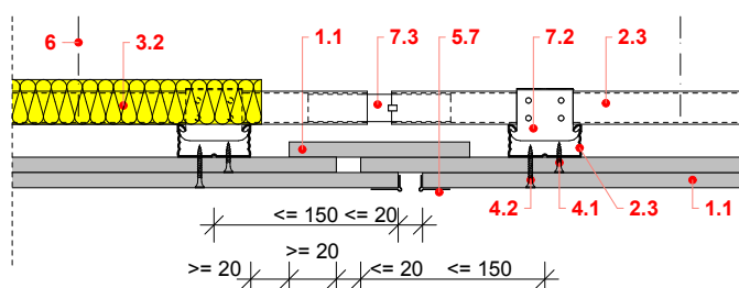
Főtartókra merőlegesen kialakított mozgási hézag; kétrétegű borítás
