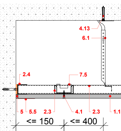
Falcsatlakozás UD-profillal
