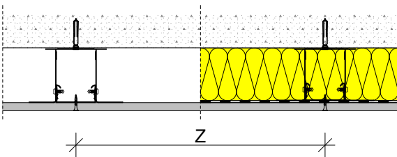
Általános részlet
