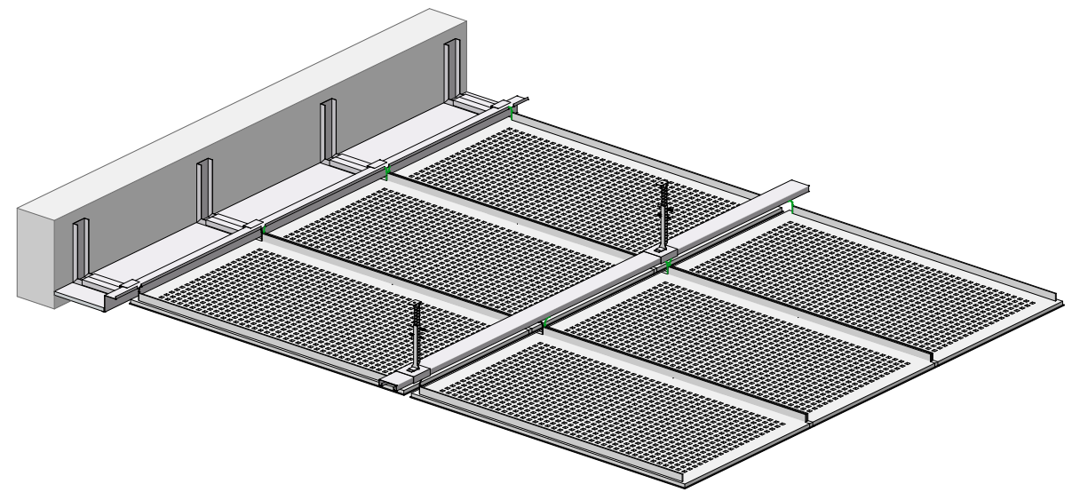
Gyptone Trap elem rögzítése a falhoz frízprofilal
