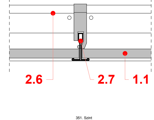
Általános részlet
