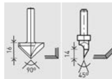
90°-os gipszkarton maró (rendelési szám: 491001) 45°-os gipszkarton maró (rendelési szám: 491000)
